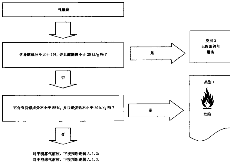
图 A.1 气溶胶的判定逻辑
