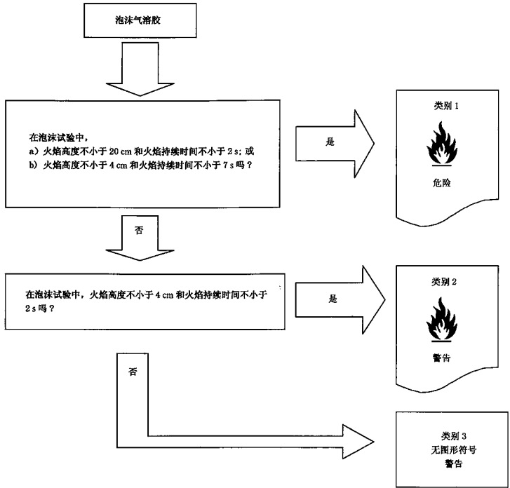
图 A.3 泡沫气溶胶判定逻辑
